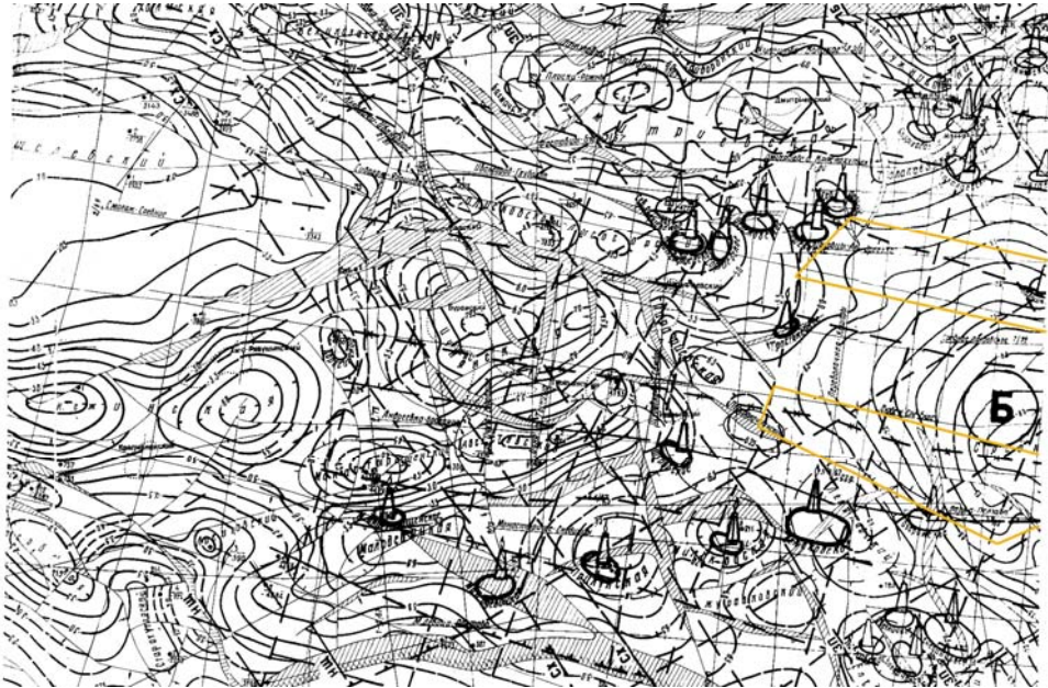
Рис. 1. Сопоставление схемы разломно-блоковой тектоники со структурной картой рельефа кристаллического фундамента (центральный грабен ДДВ на участке Ичня–Полтава).
